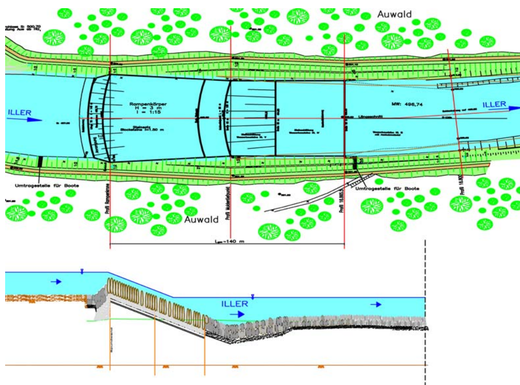
Figure 13 : Seuil en enrochements jointifs sur l'Iller.
