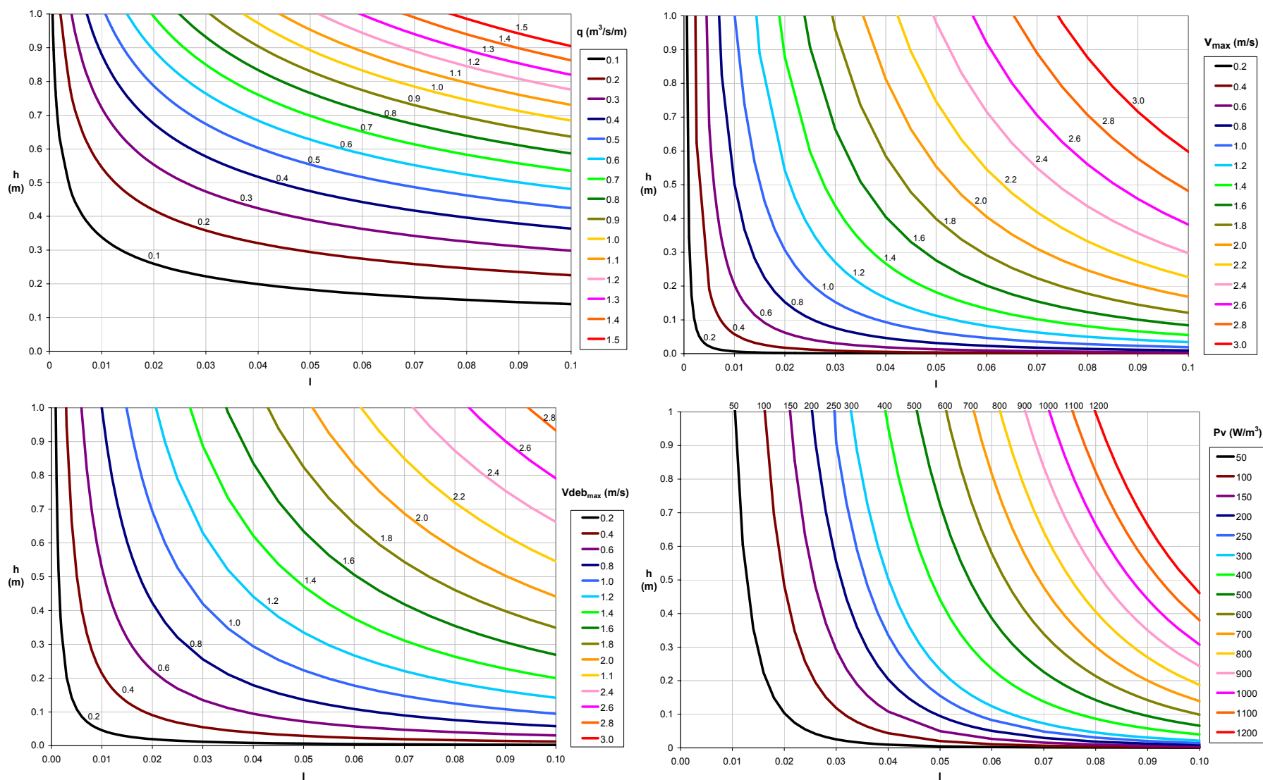
Figure A 2 : Abaque donnant q (m 3 /s/m), v_{\max} (m/s), V_{\text{deb}_{\max}} (m/s) et P_v (W/m 3 ) en fonction de h (m) et de l pour des enrochements régulièrement répartis à face arrondie à une concentration de 0.13 et D = 0.5 m
